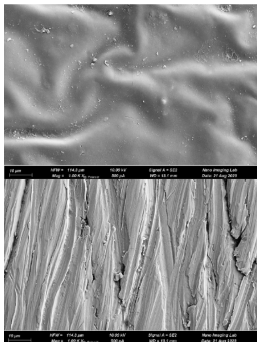
Rasterelektronenmikroskopische Aufnahmen von Standard PVC, Hochdrucklaminat (HPL), Edelstahl und Boden-PVC zeigen die unterschiedlichen Oberflächenstrukturen der verschiedenen Materialien. (Bild: A. Schneider und Nano Imaging Lab, SNI, Universität Basel)
