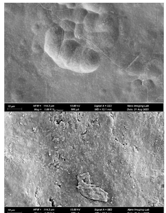
Rasterelektronenmikroskopische Aufnahmen von Standard PVC, Hochdrucklaminat (HPL), Edelstahl und Boden-PVC zeigen die unterschiedlichen Oberflächenstrukturen der verschiedenen Materialien. (Bild: A. Schneider und Nano Imaging Lab, SNI, Universität Basel)
